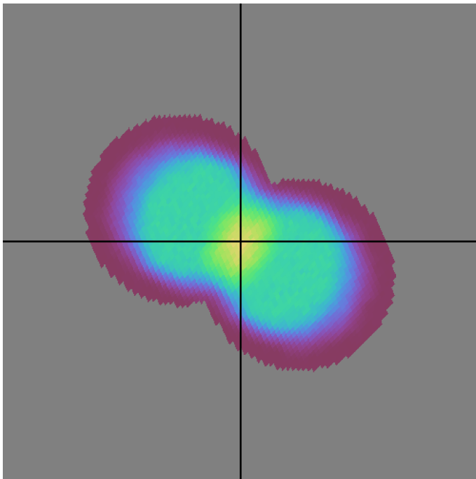
baseline_v3.0_10yrs r band: DD:EDFS NVisits
