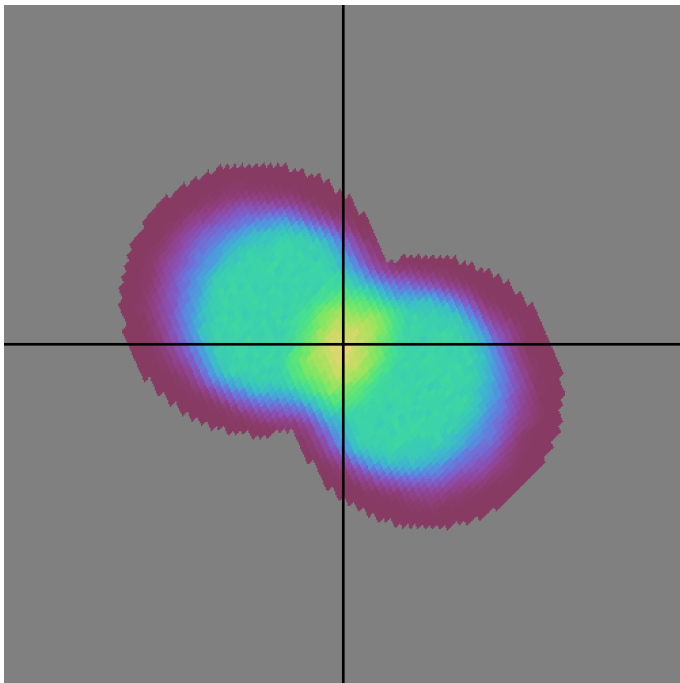
baseline_v3.0_10yrs g band: DD:EDFS NVisits
