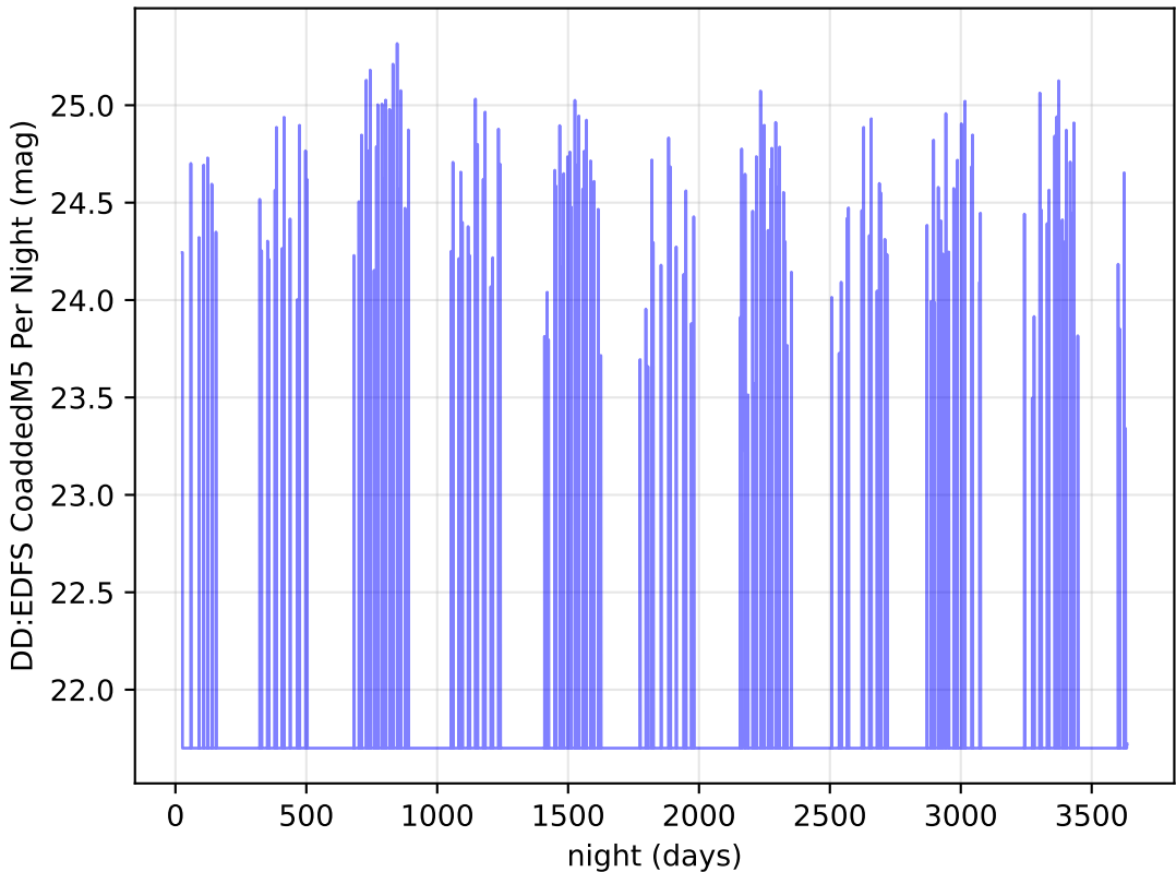
baseline_v3.0_10yrs z band: DD:EDFS CoaddedM5 Per Night
