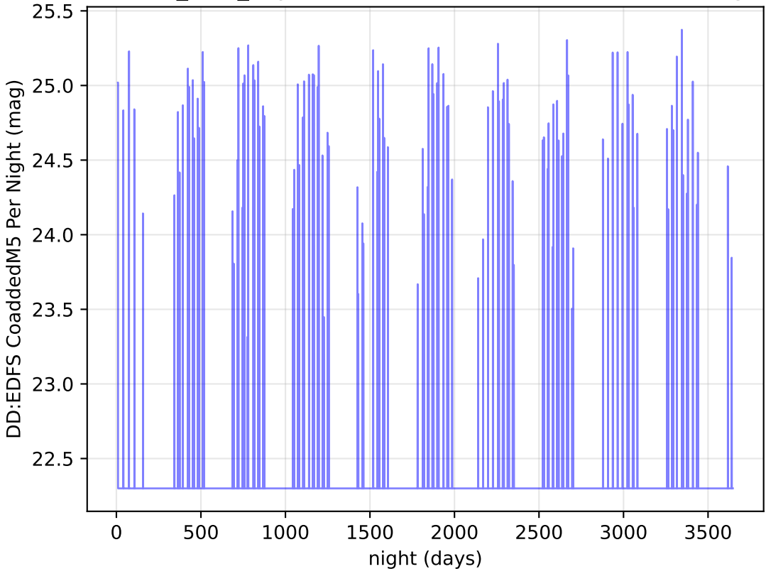
baseline_v3.0_10yrs u band: DD:EDFS CoaddedM5 Per Night
