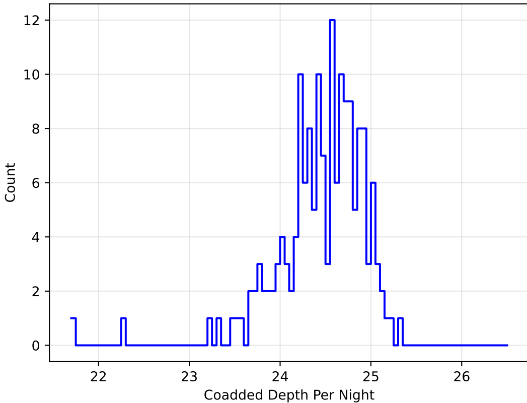
baseline_v3.0_10yrs z band: DD:EDFS CoaddM5PerNight
