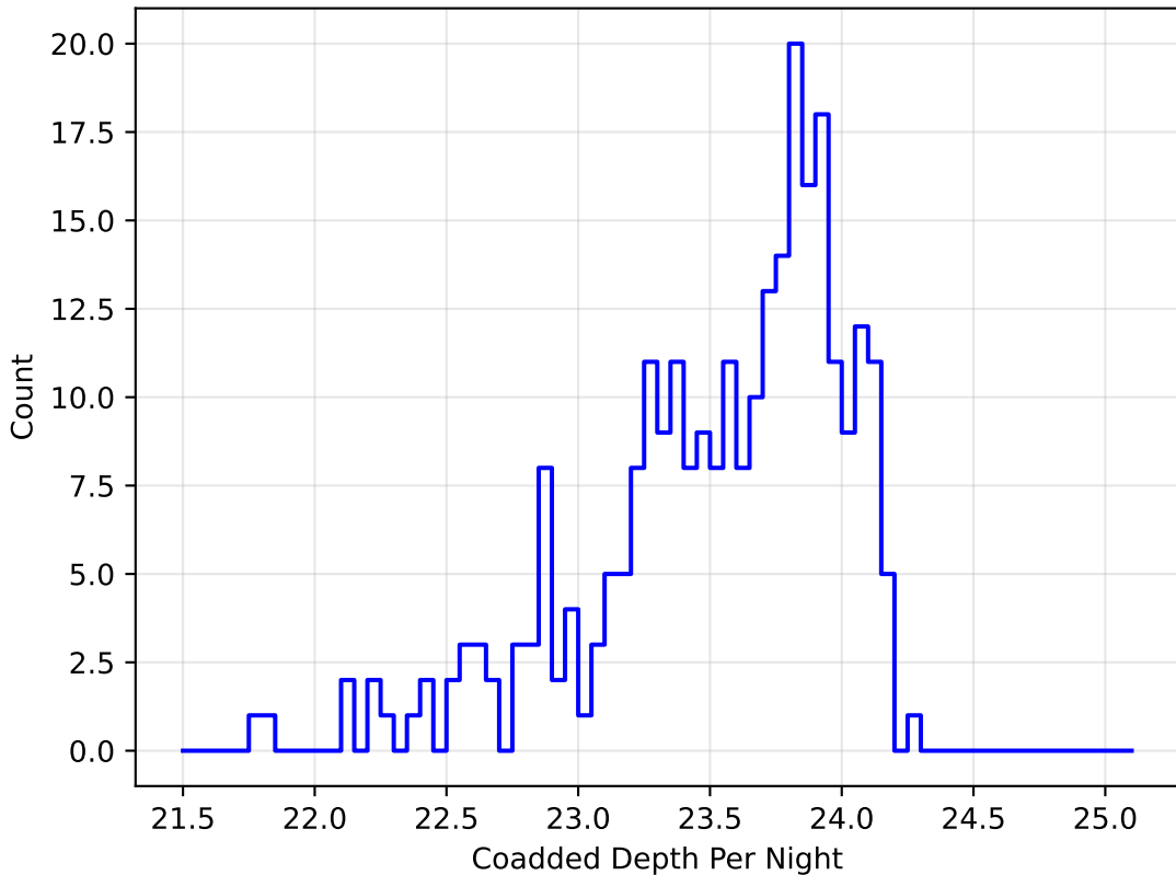
baseline_v3.0_10yrs y band: DD:EDFS CoaddM5PerNight
