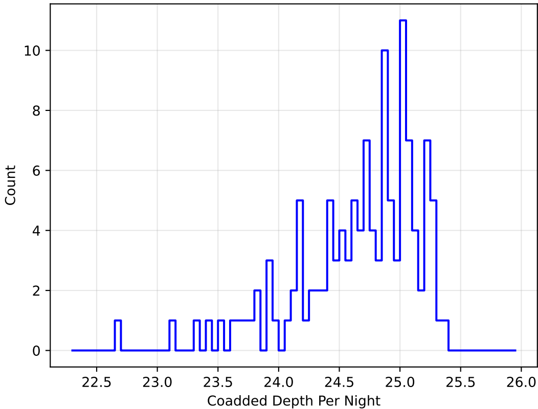
baseline_v3.0_10yrs u band: DD:EDFS CoaddM5PerNight
