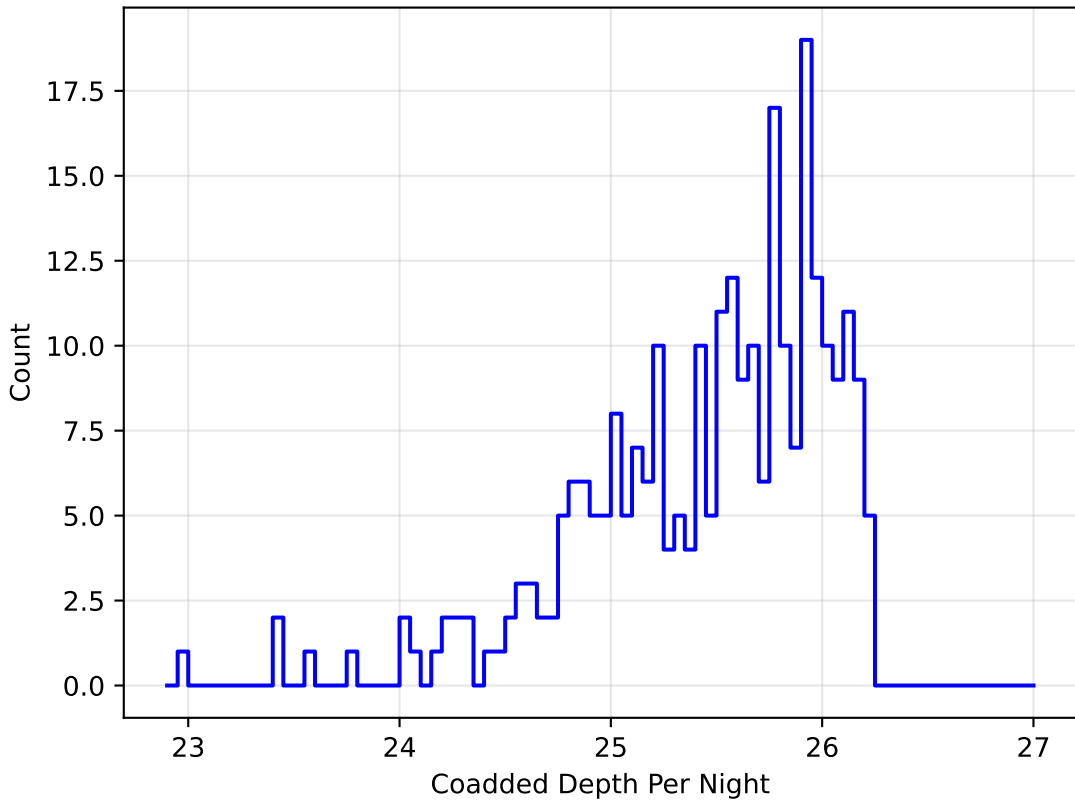
baseline_v3.0_10yrs r band: DD:EDFS CoaddM5PerNight
