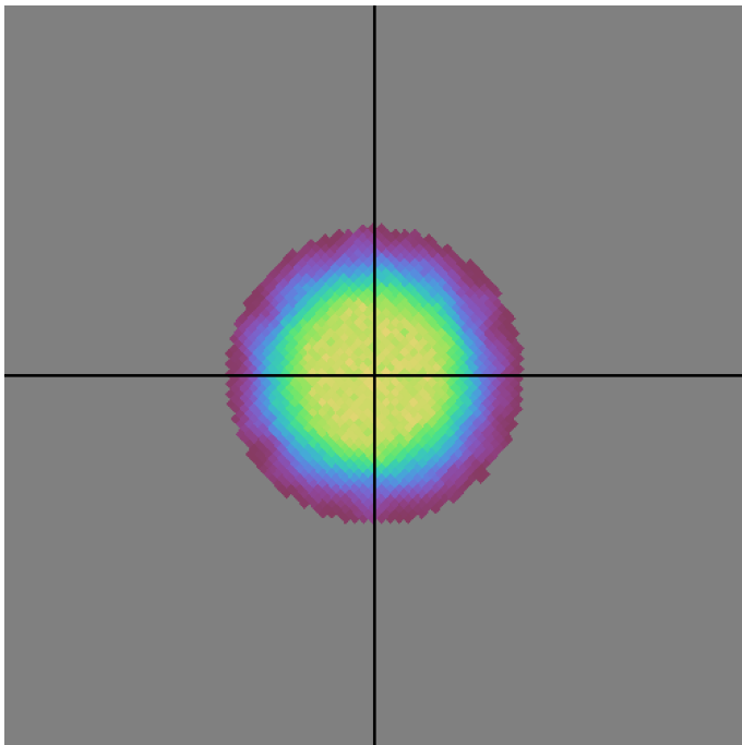
baseline_v3.0_10yrs z band: DD:ECDFS NVisits
