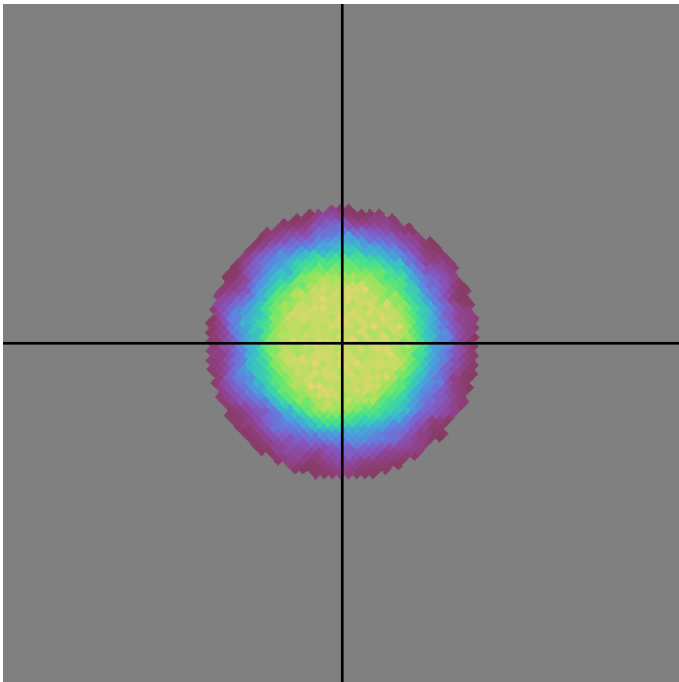
baseline_v3.0_10yrs u band: DD:ECDFS NVisits
