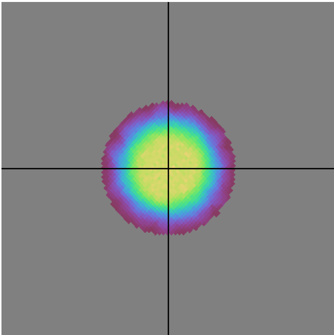
baseline_v3.0_10yrs i band: DD:ECDFS NVisits
