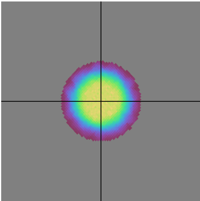
baseline_v3.0_10yrs g band: DD:ECDFS NVisits
