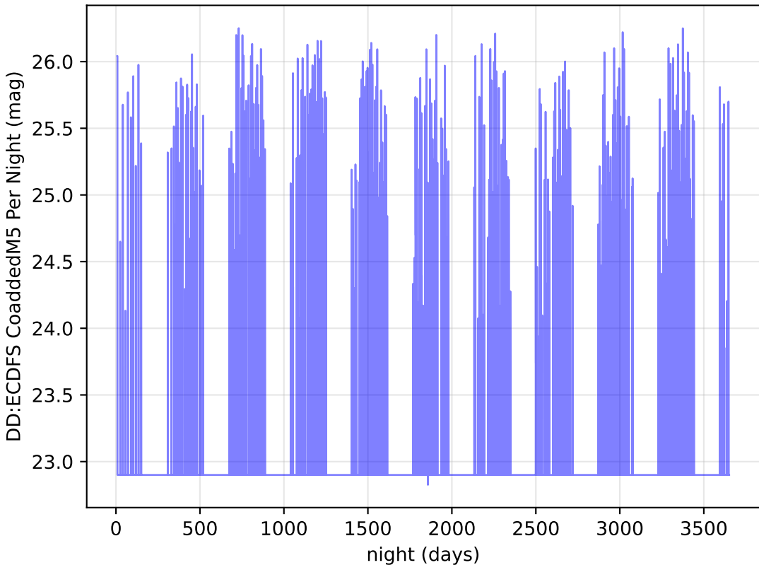
baseline_v3.0_10yrs r band: DD:ECDFS CoaddedM5 Per Night
