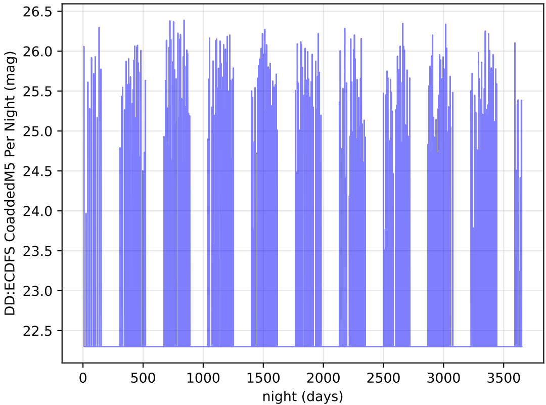
baseline_v3.0_10yrs g band: DD:ECDFS CoaddedM5 Per Night
