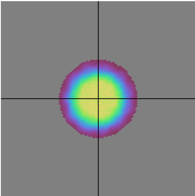
baseline_v3.0_10yrs u band: DD:COSMOS NVisits
