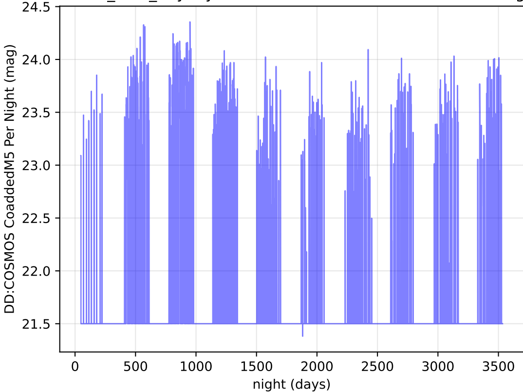
baseline_v3.0_10yrs y band: DD:COSMOS CoaddedM5 Per Night
