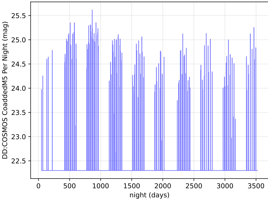
baseline_v3.0_10yrs u band: DD:COSMOS CoaddedM5 Per Night
