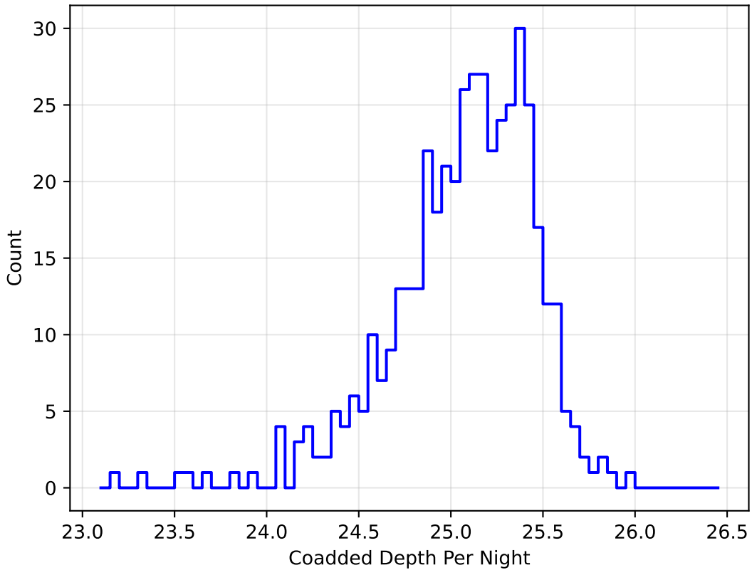
baseline_v3.0_10yrs i band: DD:COSMOS CoaddM5PerNight
