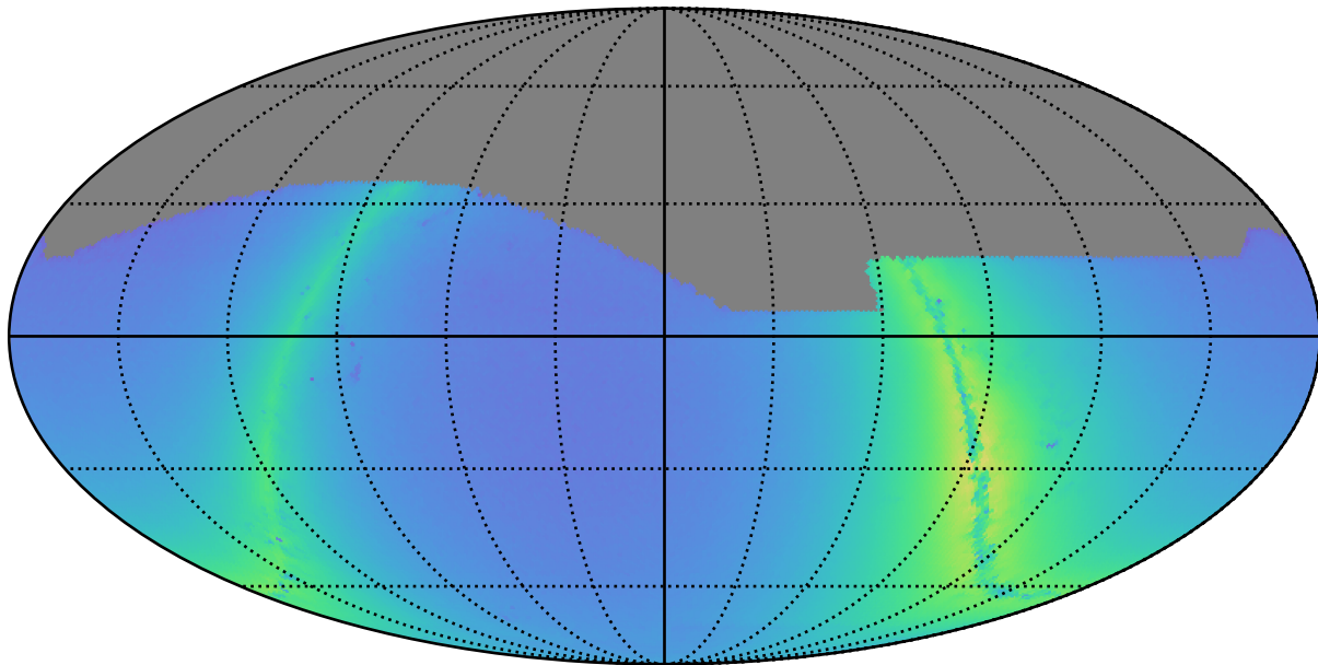
baseline_v2.1_10yrs i: Nstars_no_crowding
