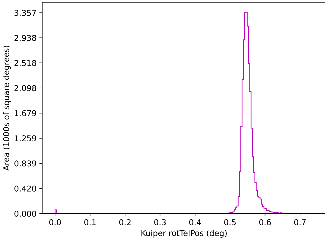
baseline_v2.1_10yrs z: Kuiper rotTelPos
