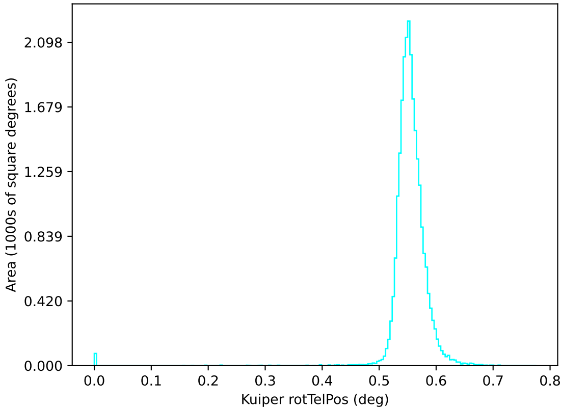
baseline_v2.1_10yrs u: Kuiper rotTelPos
