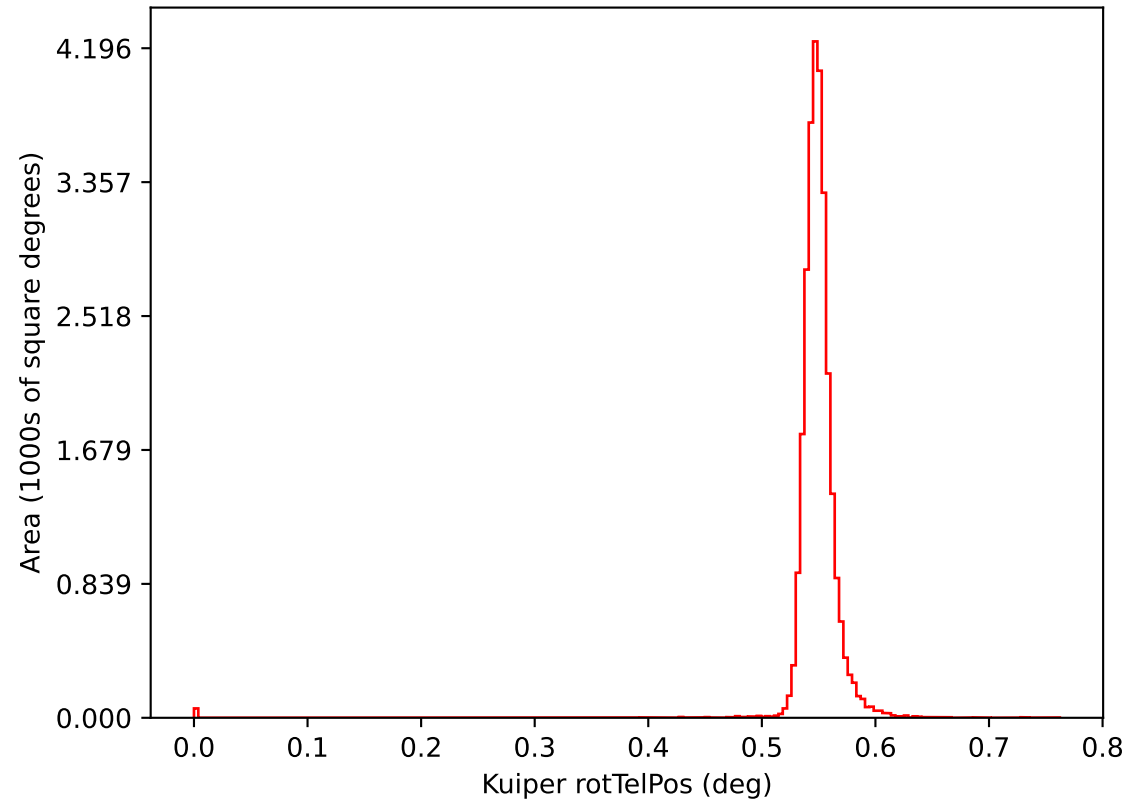
baseline_v2.1_10yrs i: Kuiper rotTelPos
