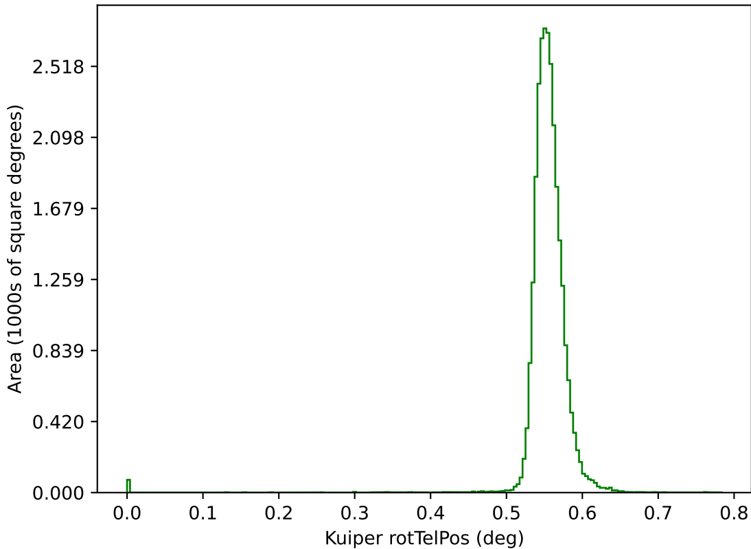
baseline_v2.1_10yrs g: Kuiper rotTelPos
