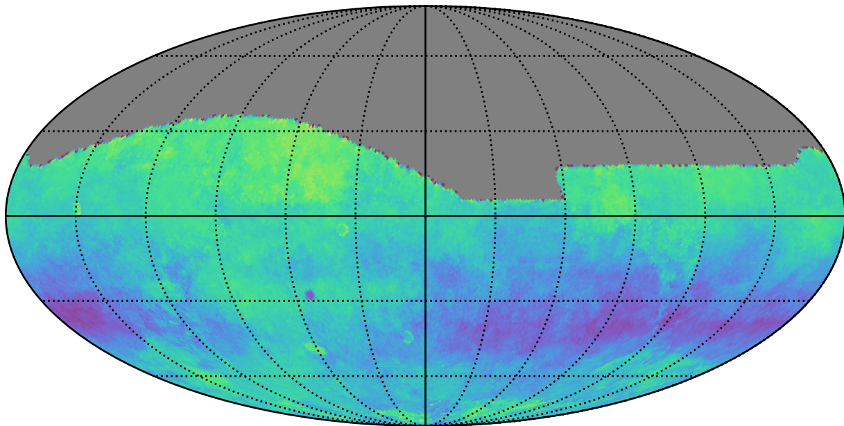
baseline_v2.1_10yrs z: Kuiper rotSkyPos
