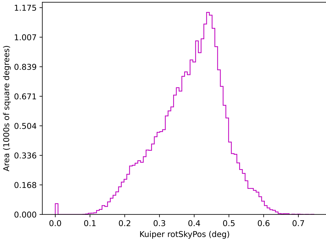
baseline_v2.1_10yrs z: Kuiper rotSkyPos
