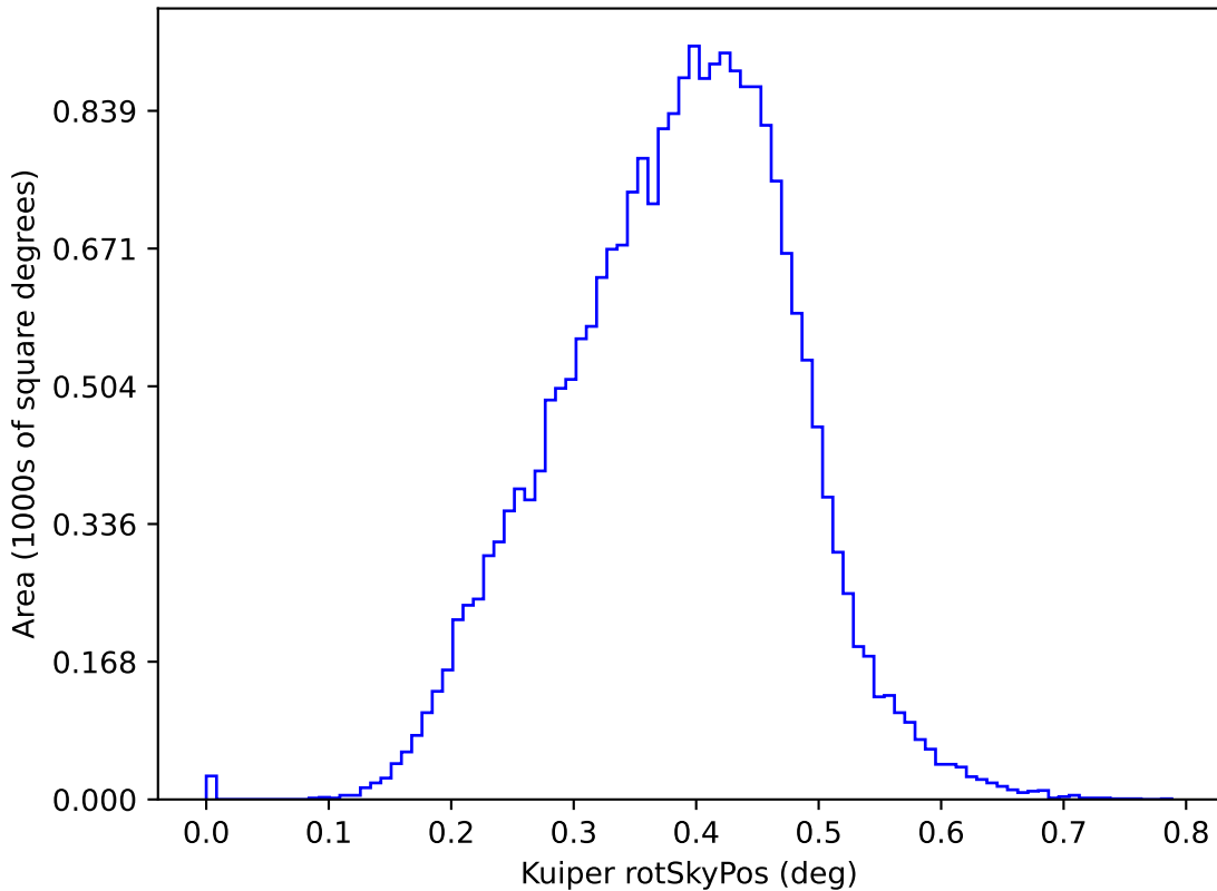
baseline_v2.1_10yrs y: Kuiper rotSkyPos
