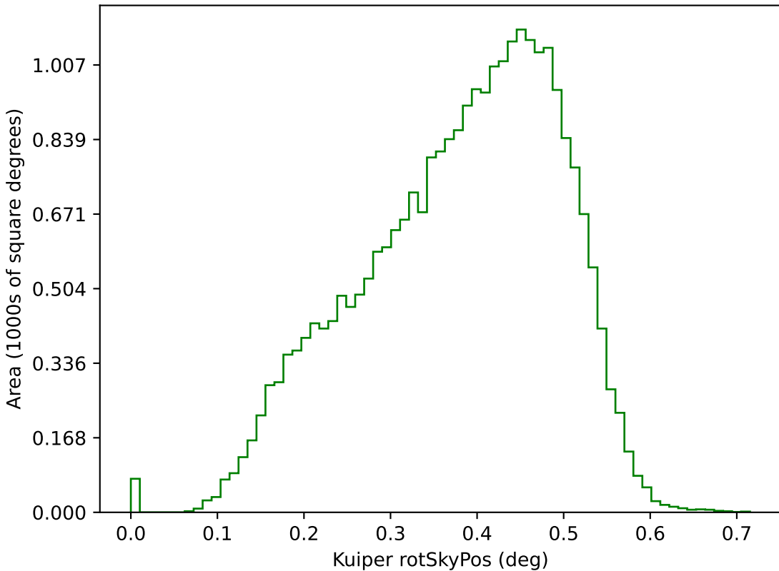
baseline_v2.1_10yrs g: Kuiper rotSkyPos
