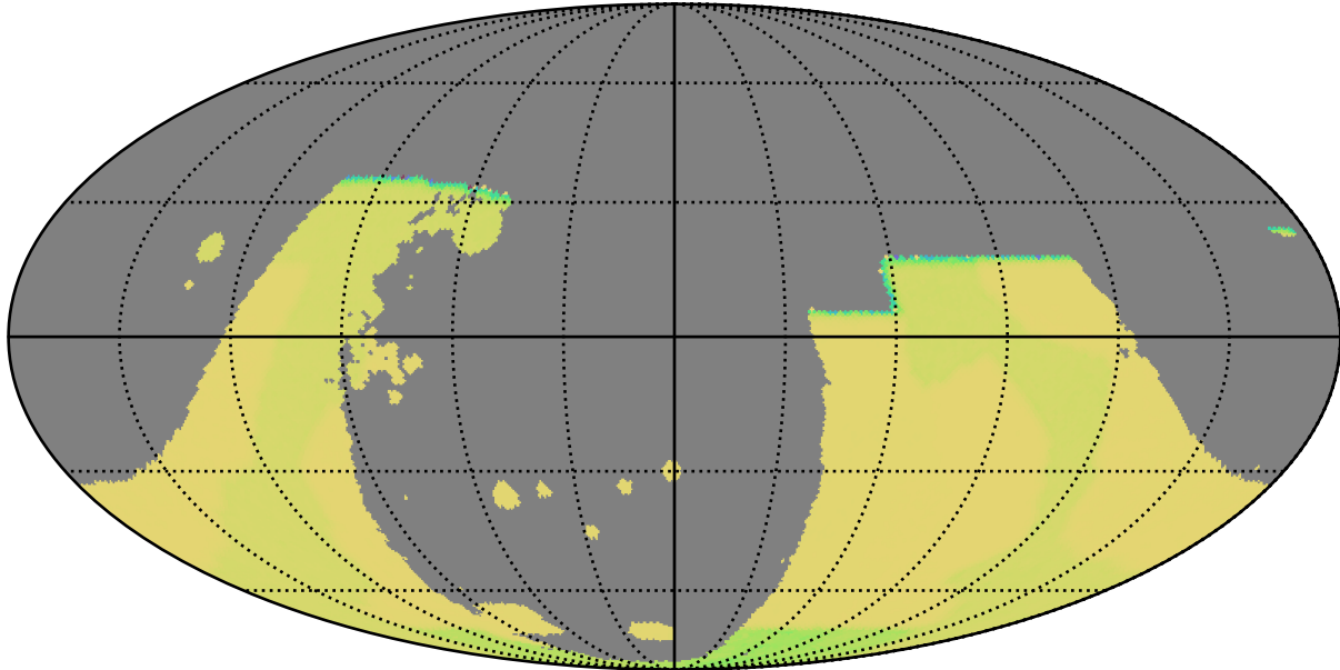
baseline_v2.1_10yrs : GalPlaneVisitIntervalsTimescales_combined_map_Tau_46_5
