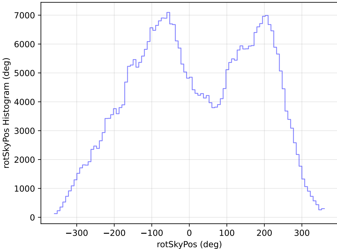
baseline_v2.1_10yrs All sky y band: rotSkyPos Histogram
