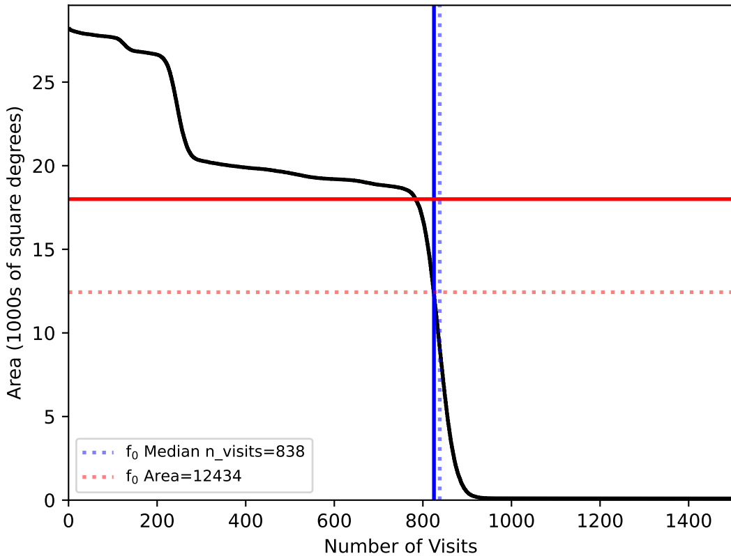
baseline_v2.1_10yrs All sky: f0
