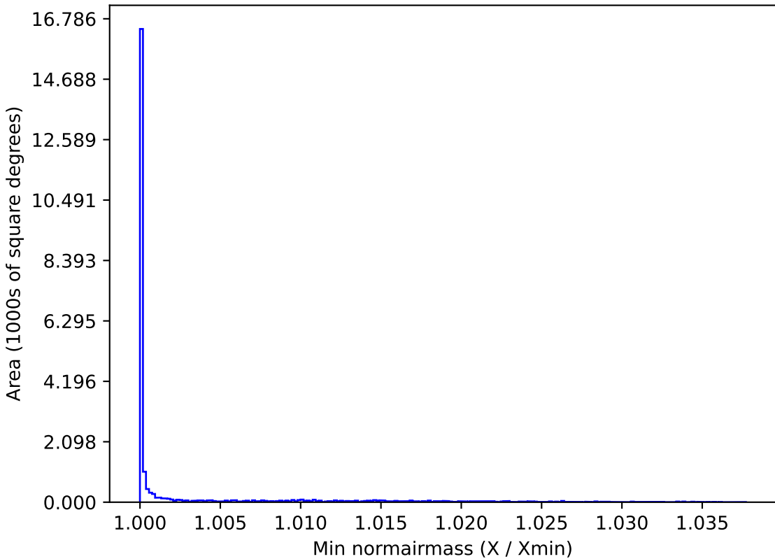
baseline_v2.1_10yrs All sky y band: Min normairmass
