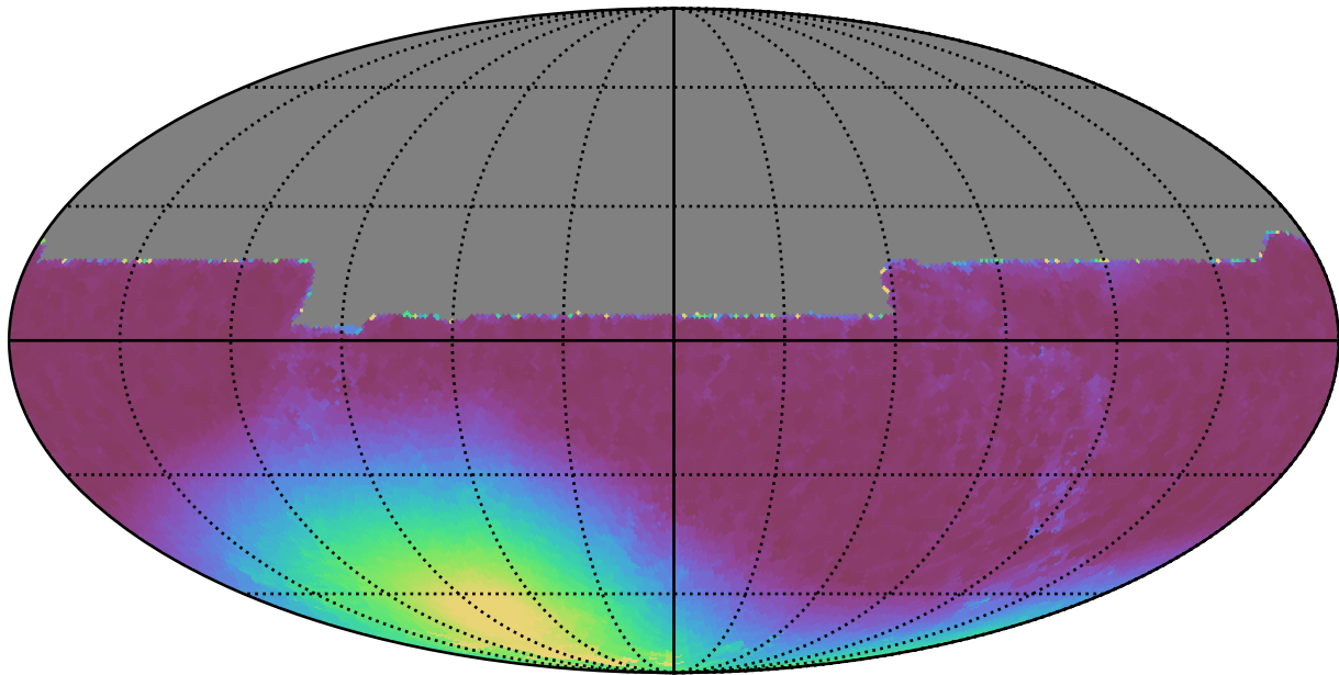
baseline_v2.1_10yrs All sky y band: Min moonDistance
