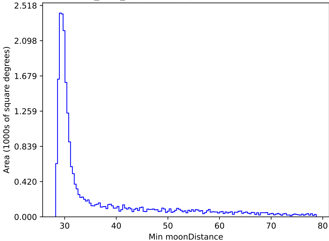
baseline_v2.1_10yrs All sky y band: Min moonDistance
