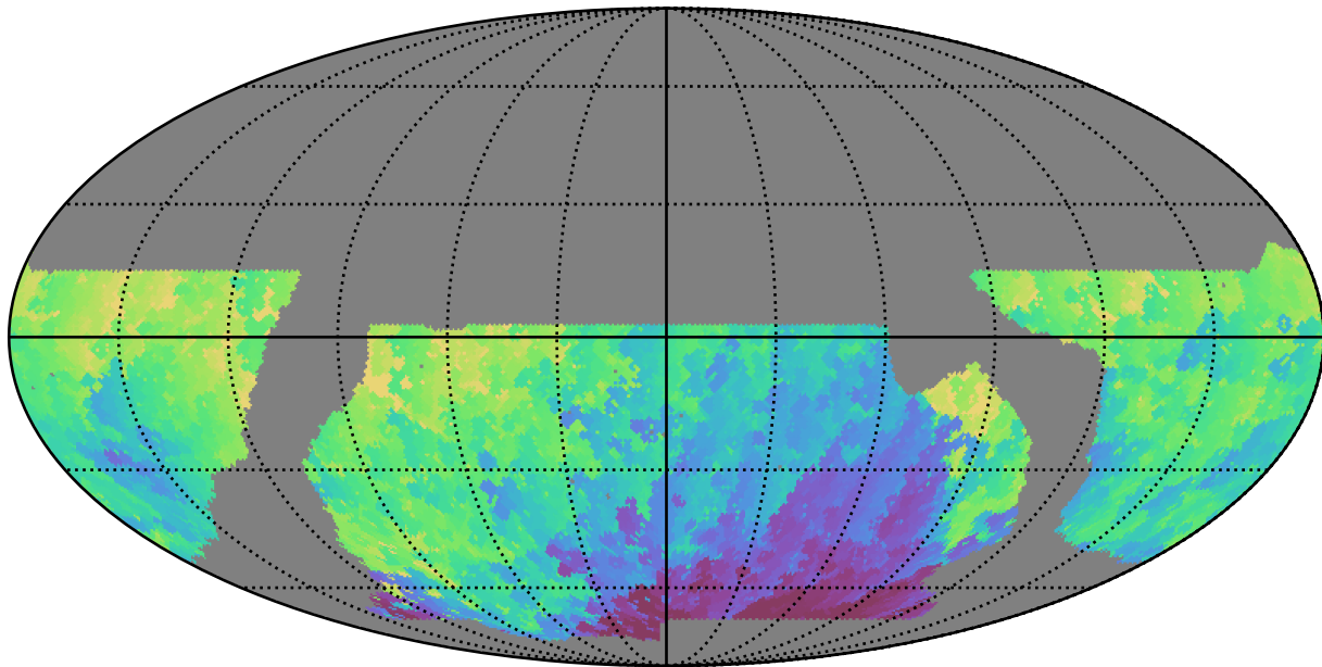
baseline_v2.1_10yrs WFD y band: Min HA
