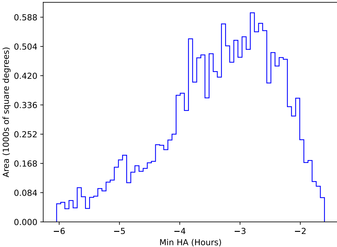
baseline_v2.1_10yrs WFD y band: Min HA
