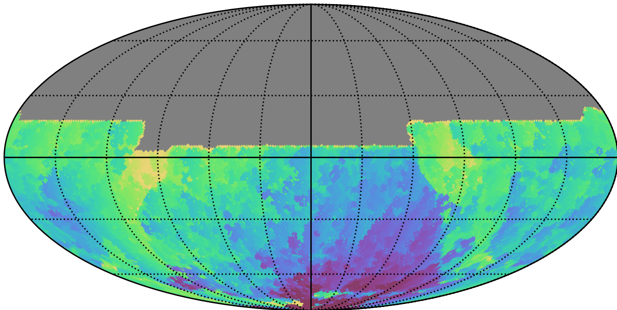
baseline_v2.1_10yrs All sky y band: Min HA
