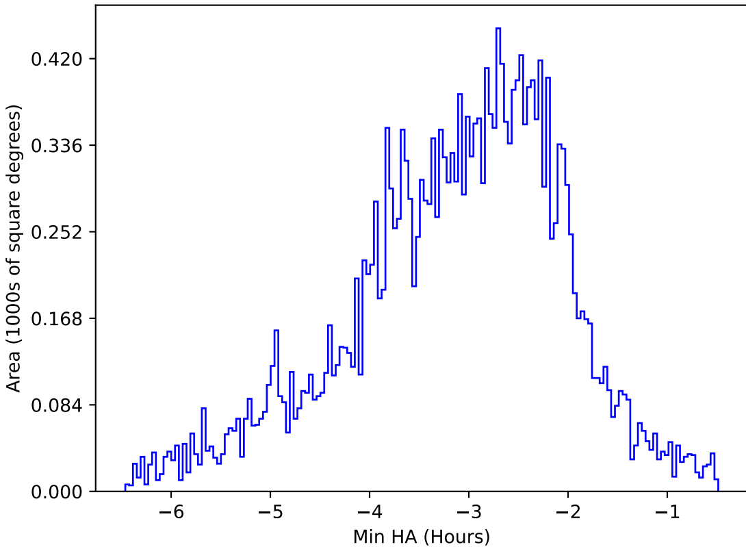
baseline_v2.1_10yrs All sky y band: Min HA
