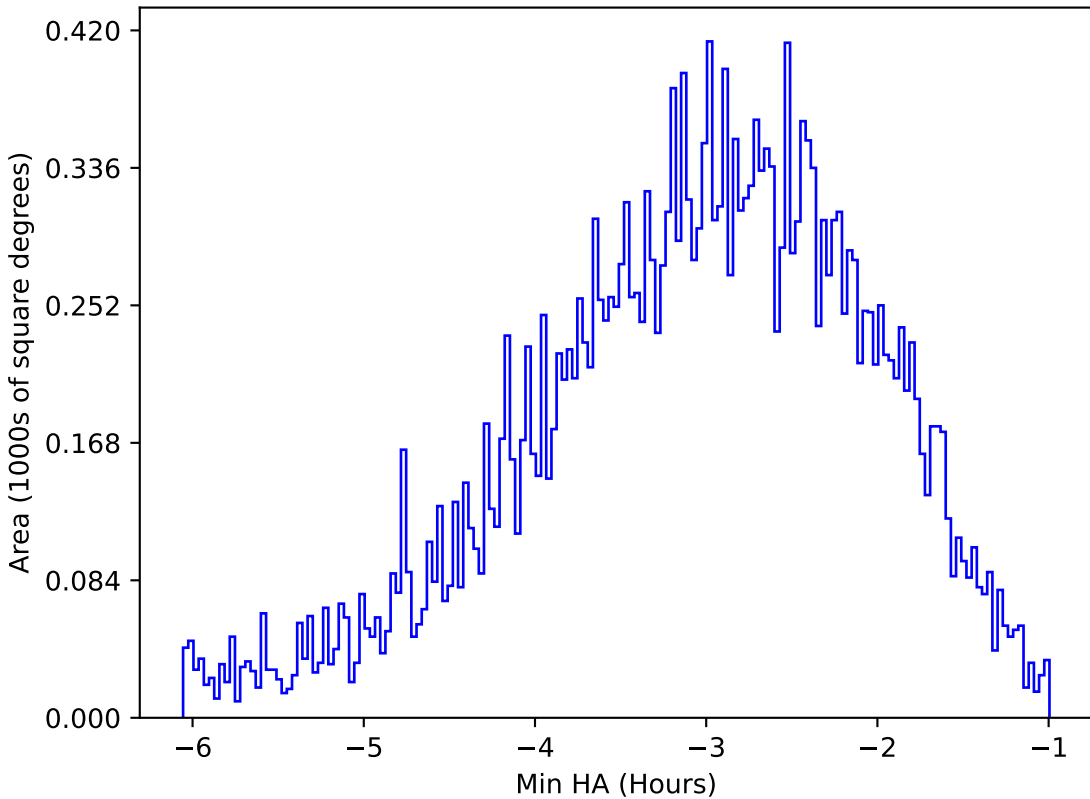
baseline_v2.1_10yrs All sky i band: Min HA
