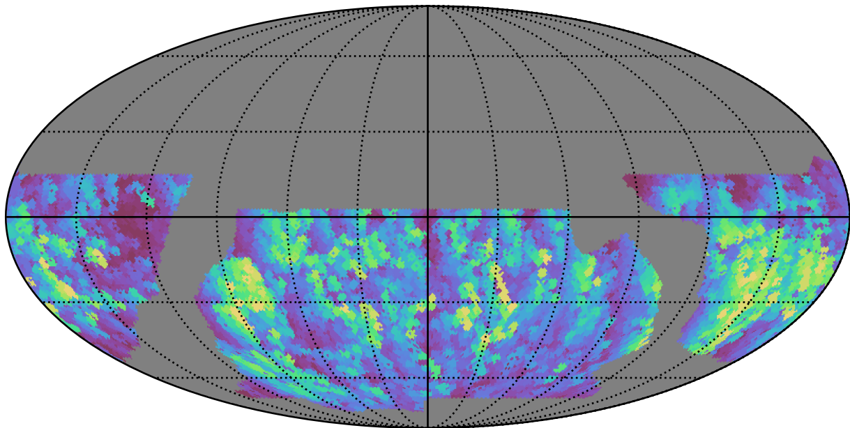
baseline_v2.1_10yrs WFD y band: Max normairmass
