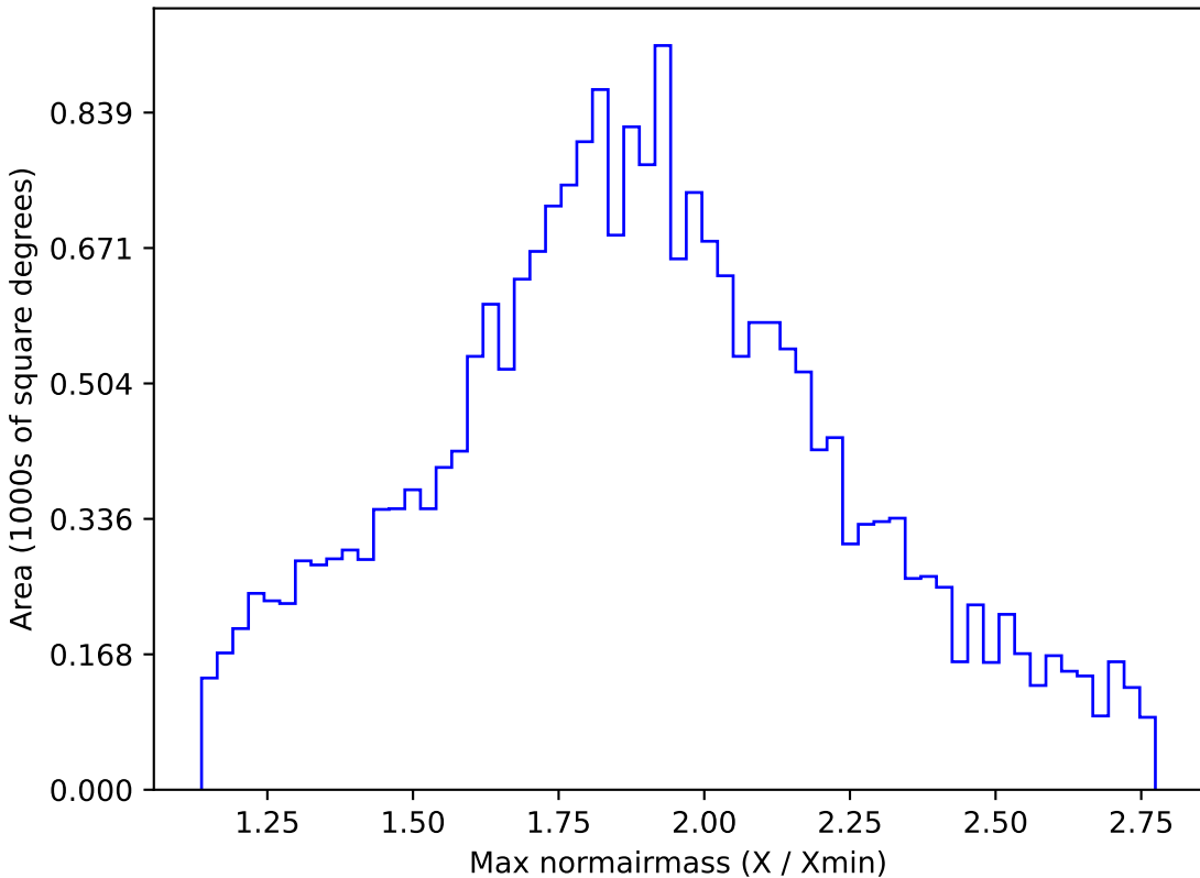
baseline_v2.1_10yrs All sky y band: Max normairmass
