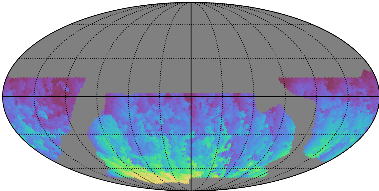
baseline_v2.1_10yrs WFD y band: Max HA
