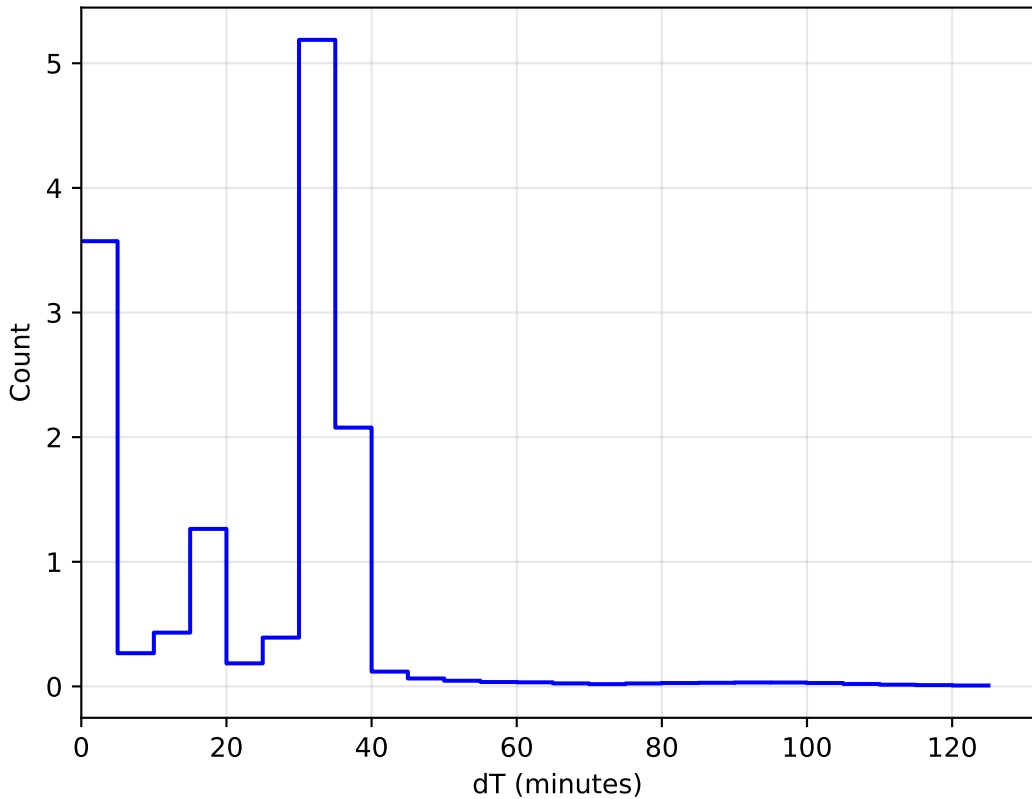
1e6 baseline_v2.1_10yrs All sky: DeltaT Histogram
