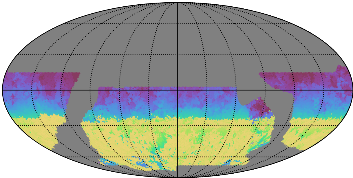
baseline_v2.1_10yrs WFD y band: AngleRange rotSkyPos
