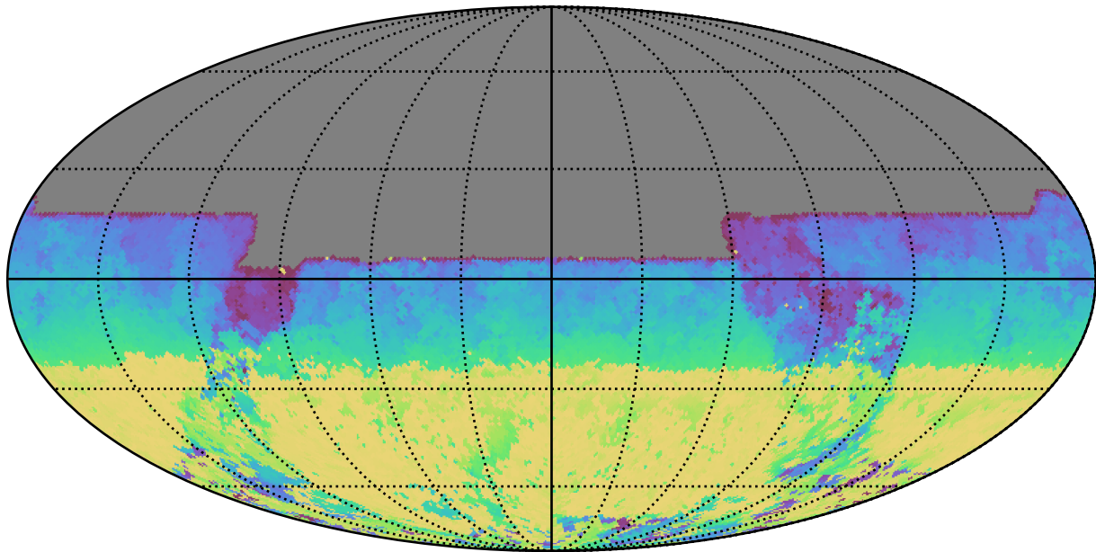
baseline_v2.1_10yrs All sky y band: AngleRange rotSkyPos
