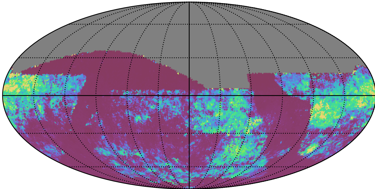
baseline_v2.1_10yrs All sky iz bands: 75th Percentile Intranight Timespan
