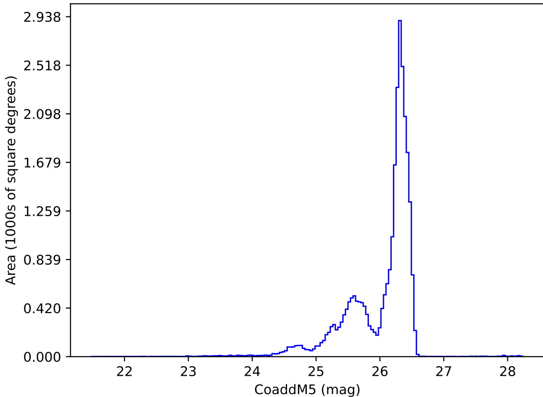
baseline_v2.1_10yrs i: CoaddM5
