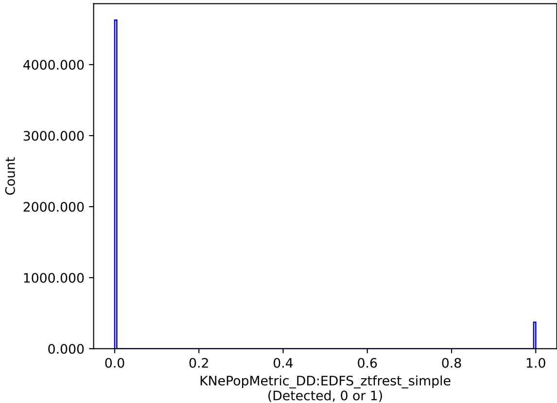
baseline_v2.1_10yrs DD:EDFS: KNePopMetric_DD:EDFS_ztfrest_simple
