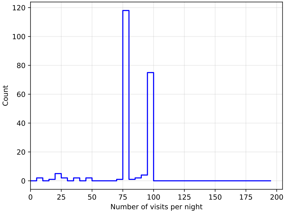
baseline_v2.1_10yrs all bands: DD:ELAISS1 NVisitsPerNight
