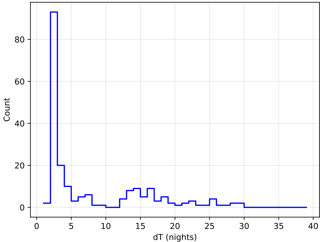
baseline_v2.1_10yrs all bands: DD:ELAISS1 Delta Nights Histogram
