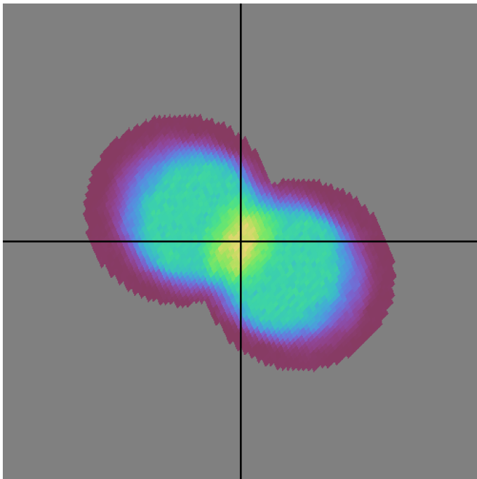
baseline_v2.1_10yrs r band: DD:EDFS NVisits
